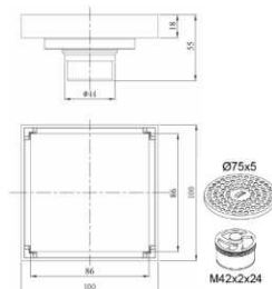
HMS 05 CH Floor Drainer • Material : Brass • Usage : Long-term use • Polished : Chrome Rp. 300.000
